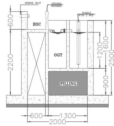
SECTION D-D
